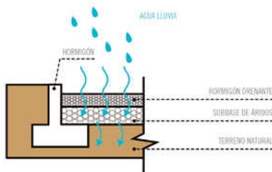
FIG.10. PAVIMENTO PERMEABLE CON INFILTRACIÓN
