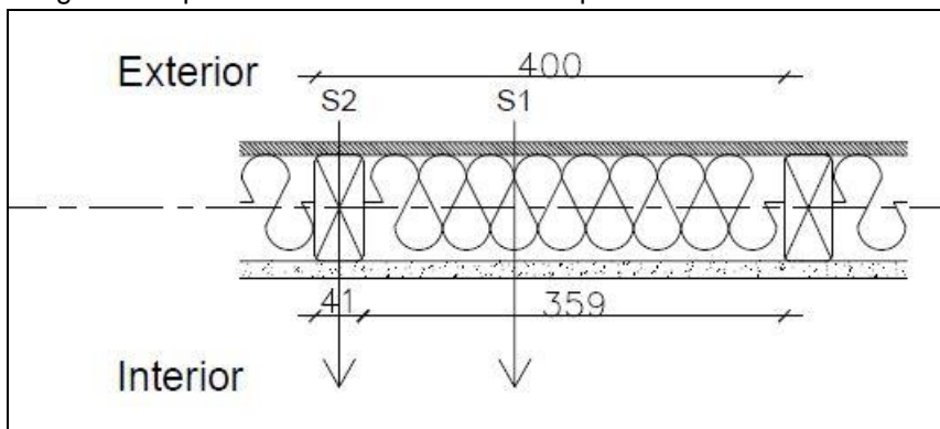
Imagen 1. Representación de una sección tipo de los sectores en muro 41x90mm (2x4) @ 40cm
