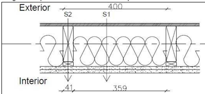
Imagen 1. Representación de una sección tipo de los sectores en muro 41x138mm (2x6) @ 40cm
