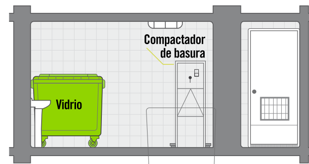
Corte A-A'
