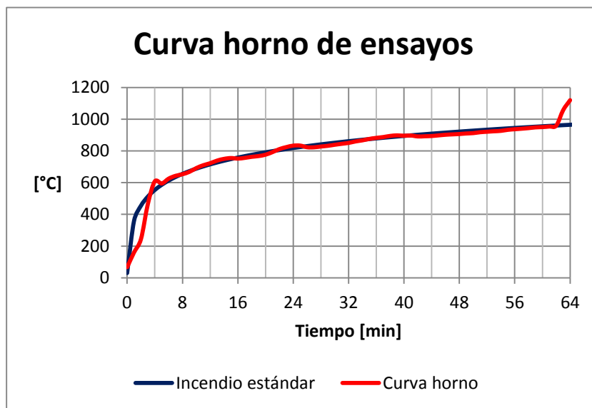
Figura 6.1 Temperatura promedio horno de ensayo
