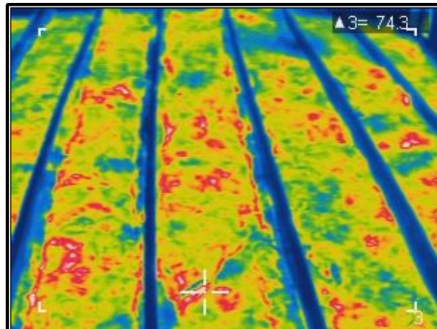
Figura 6.3 Imagen termográfica a los 35 minutos de ensayo
