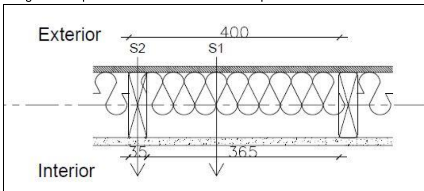
Imagen 1. Representación de una sección tipo de los sectores en muro 35x124mm (2x5) @ 40cm
