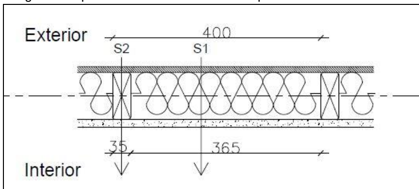
Imagen 1. Representación de una sección tipo de los sectores en muro 35x90mm (2x4) @ 40cm
