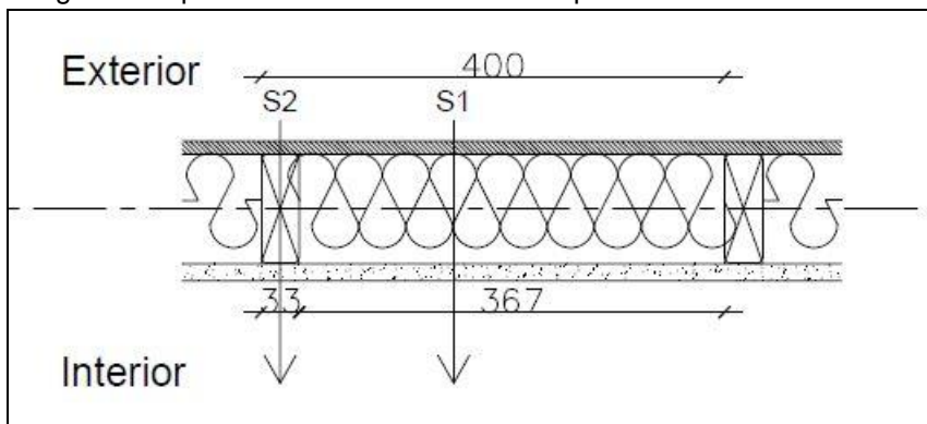
Imagen 1. Representación de una sección tipo de los sectores en muro 33x94mm (2x4) @ 40cm
