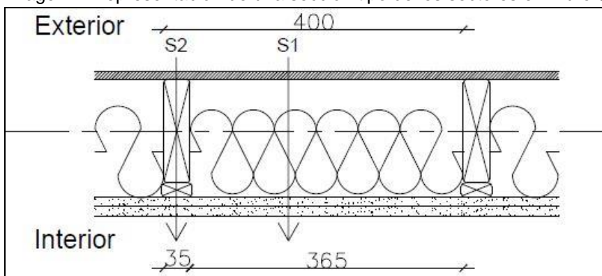
Imagen 1. Representación de una sección tipo de los sectores en muro 35x138mm (2x6) @ 40cm
