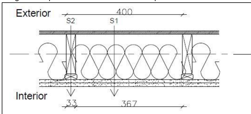
Imagen 1. Representación de una sección tipo de los sectores en muro 33x138mm (2x6) @ 40cm
