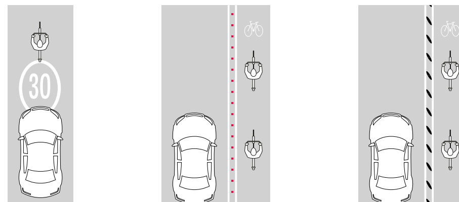
FIGURA 18. ESQUEMAS DE SEGREGACIÓN, SEGÚN VELOCIDADES DE CIRCULACIÓN.
