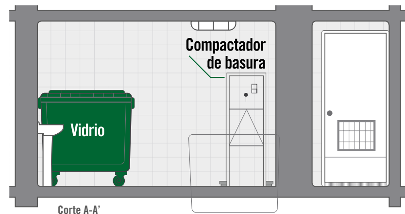
FIGURA 15. PLANTA DE RECINTO PARA LA GESTIÓN DE RESIDUOS (RGRD), DE REFERENCIA.
