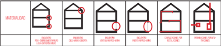
FIGURA 13. ENCUENTROS Y PERFORACIONES DONDE SE PRODUCEN INFILTRACIONES.
