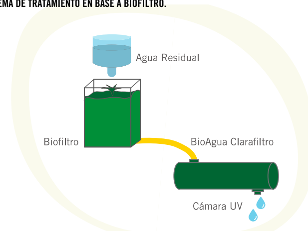
FIGURA 22. SISTEMA DE TRATAMIENTO EN BASE A BIOFILTRO.
