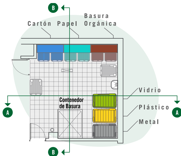
FIGURA 14. PLANTA DE RECINTO PARA LA GESTIÓN DE RESIDUOS (RGRD), DE REFERENCIA.
