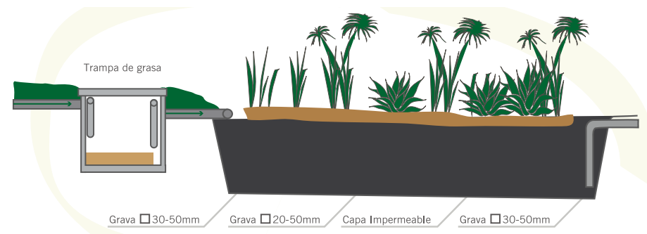
FIGURA 20. SISTEMA FILTRO JARDINERA.
